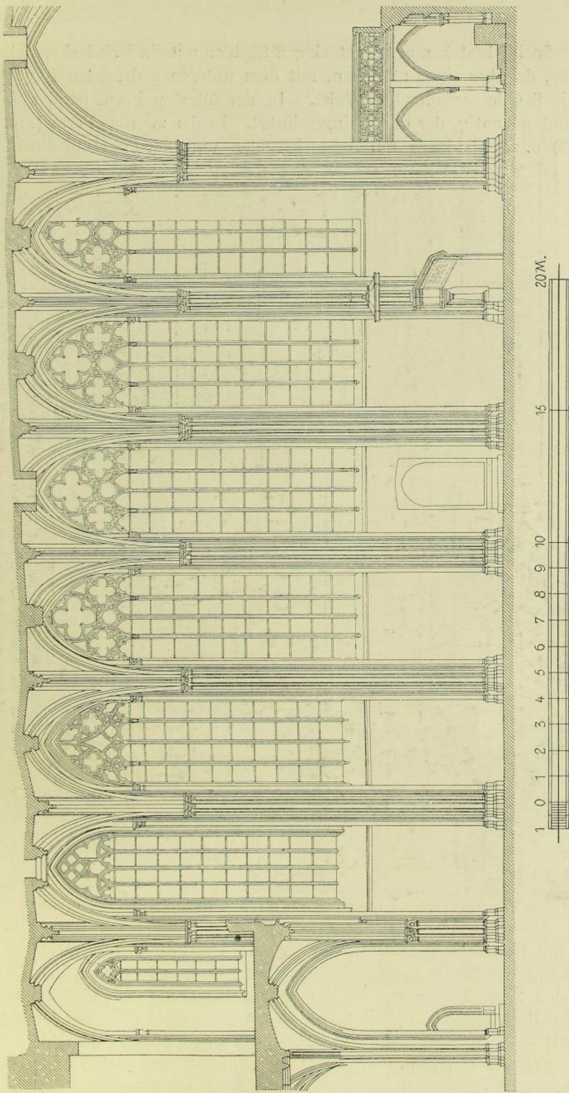
Fig. 190. Längsschnitt durch das Mittelschiff des Langhauses, Ansicht gegen Norden (Meßbildaufnahme).
