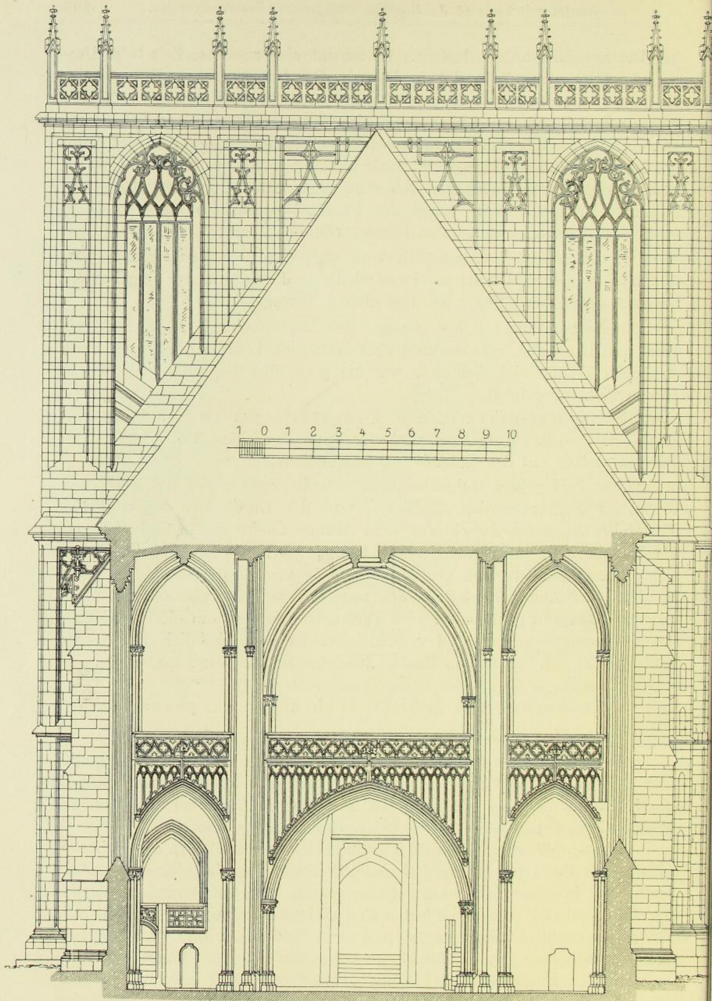
Fig. 223. Schnitt durch das Langhaus, Blick nach Westen (mit den 1869 erbauten Emporen im Süd- und Hauptschiff). Meßbildaufnahme.
