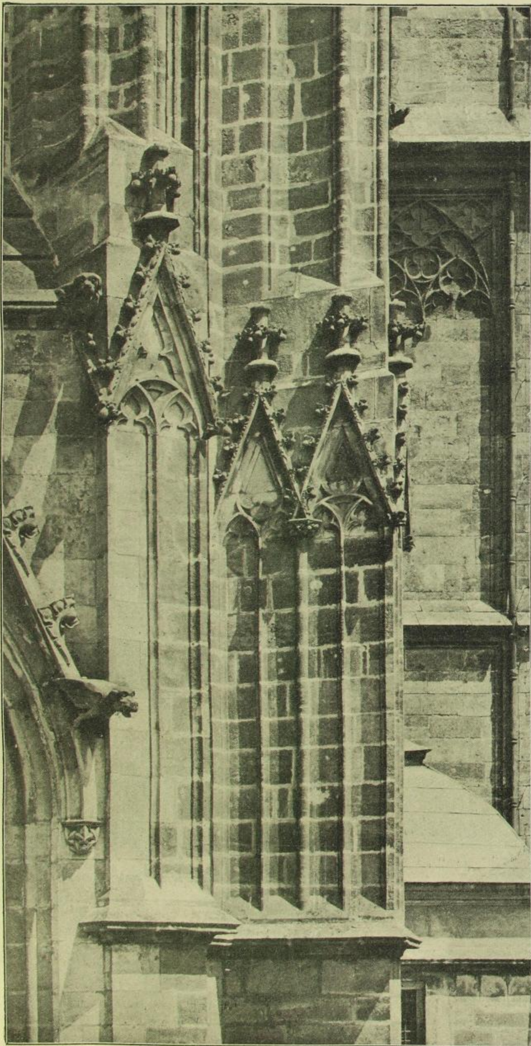
Fig. 259. Fürstencapelle, unterer Teil der westlichen Strebepfeiler,
