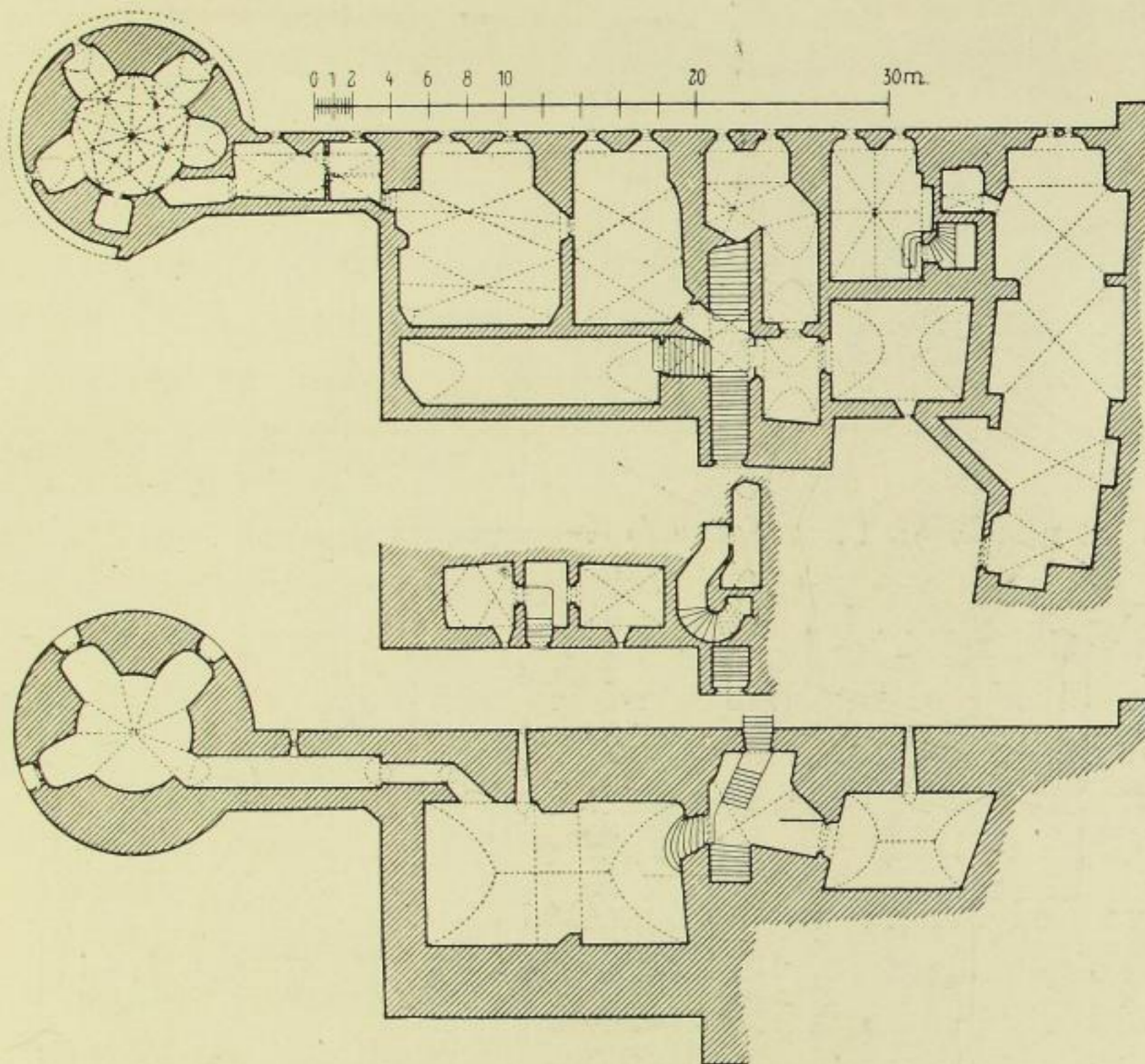
Fig. 443. Bischofsschloß, Grundriß der drei Kellergeschosse.
