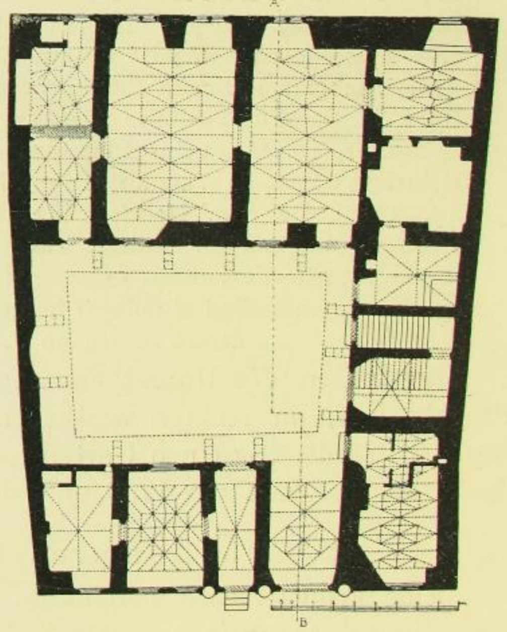
Fig. 480. Dompropstei, Grundriß des Erdgeschosses.
