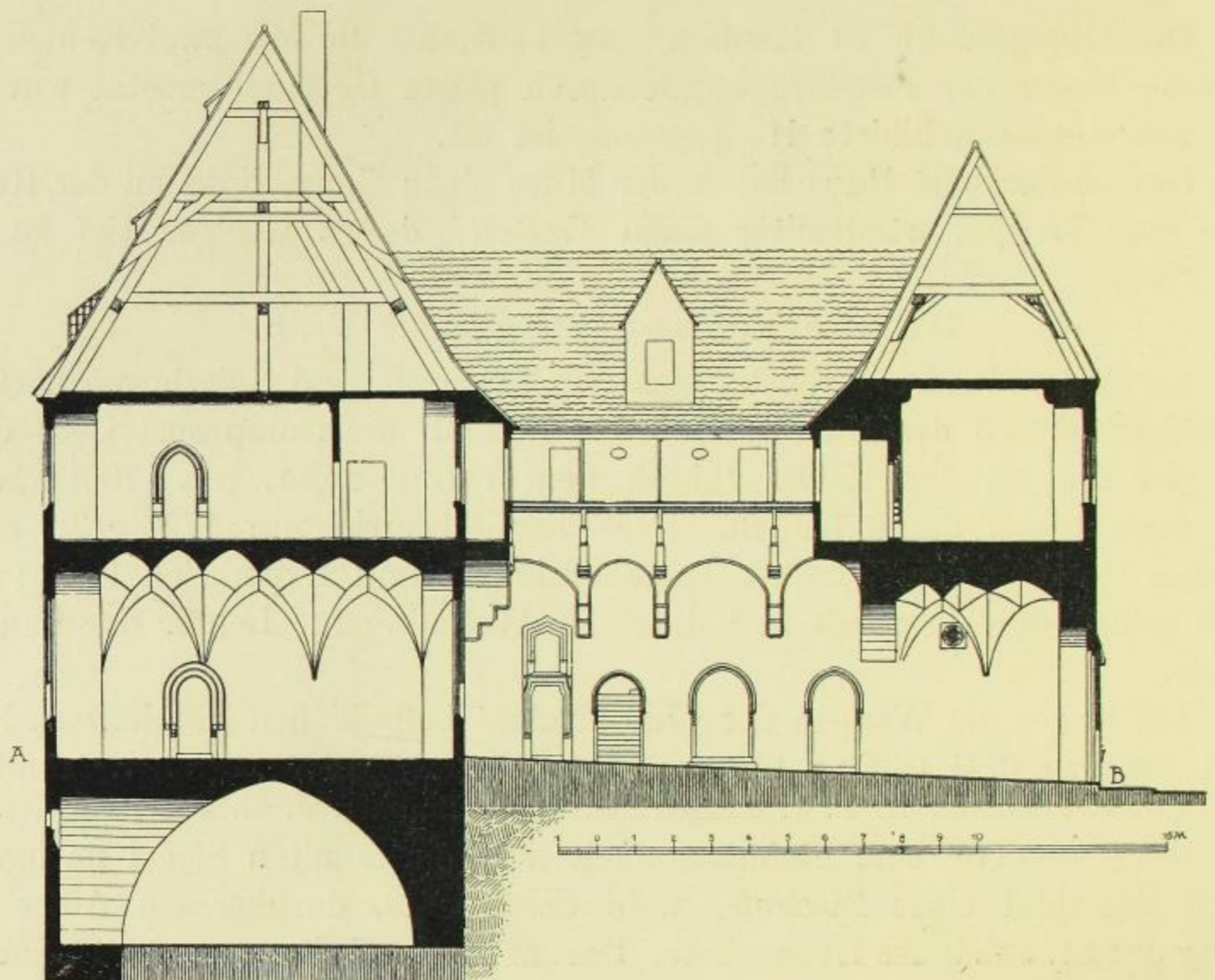
Fig. 478. Dompropstei, Querschnitt.
