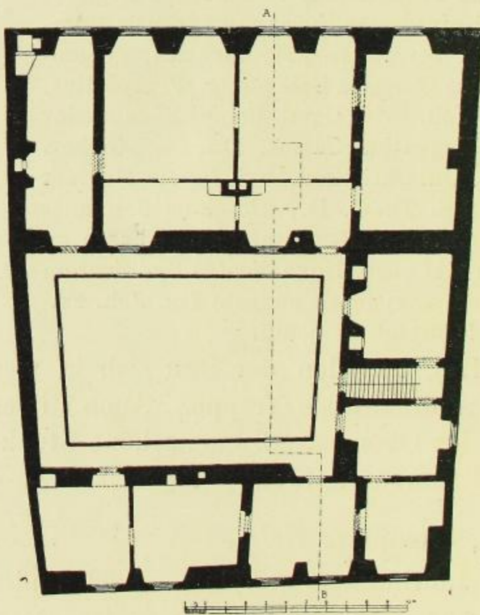
Fig. 479. Dompropstei, Grundriß des Obergeschosses.
