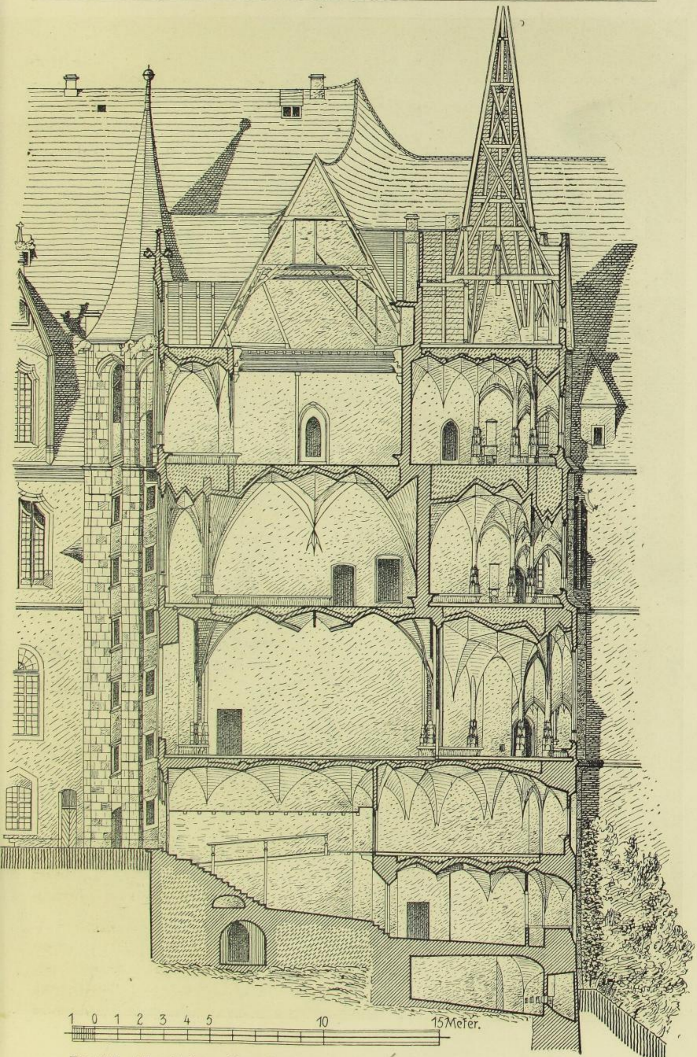
Fig. 506. Albrechtsburg. Querschnitt durch den Südbau, nach der Aufnahme von 1839
