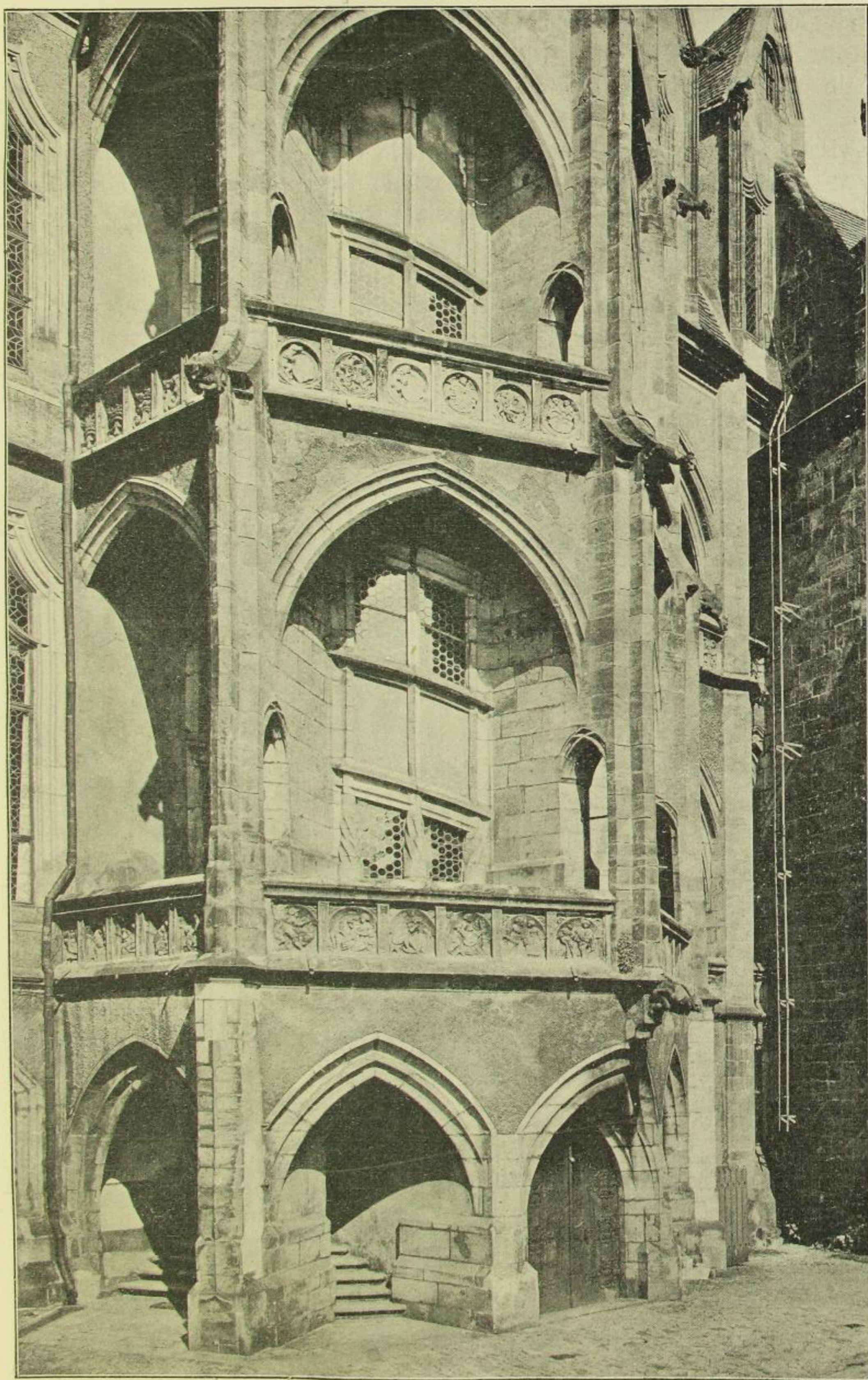
Fig. 538. Albrechtsburg, Großer Wendelstein, Ansicht von Westen.
