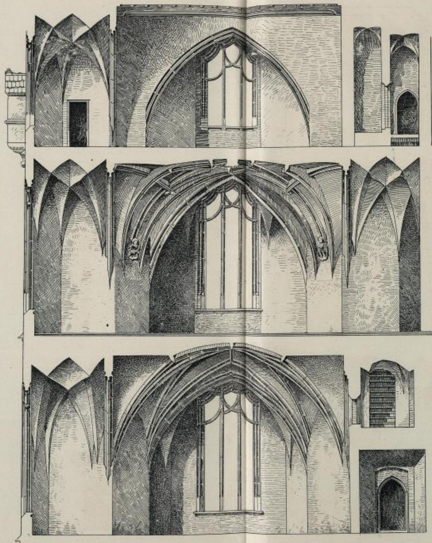
Albrechtsburg, Nordostturm, Schnitt durch die drei oberen Geschosse.
