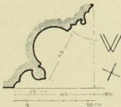
Fig. 596. Dom, Westfenster im Untergeschoß des Nordwestturmes, Profil.
