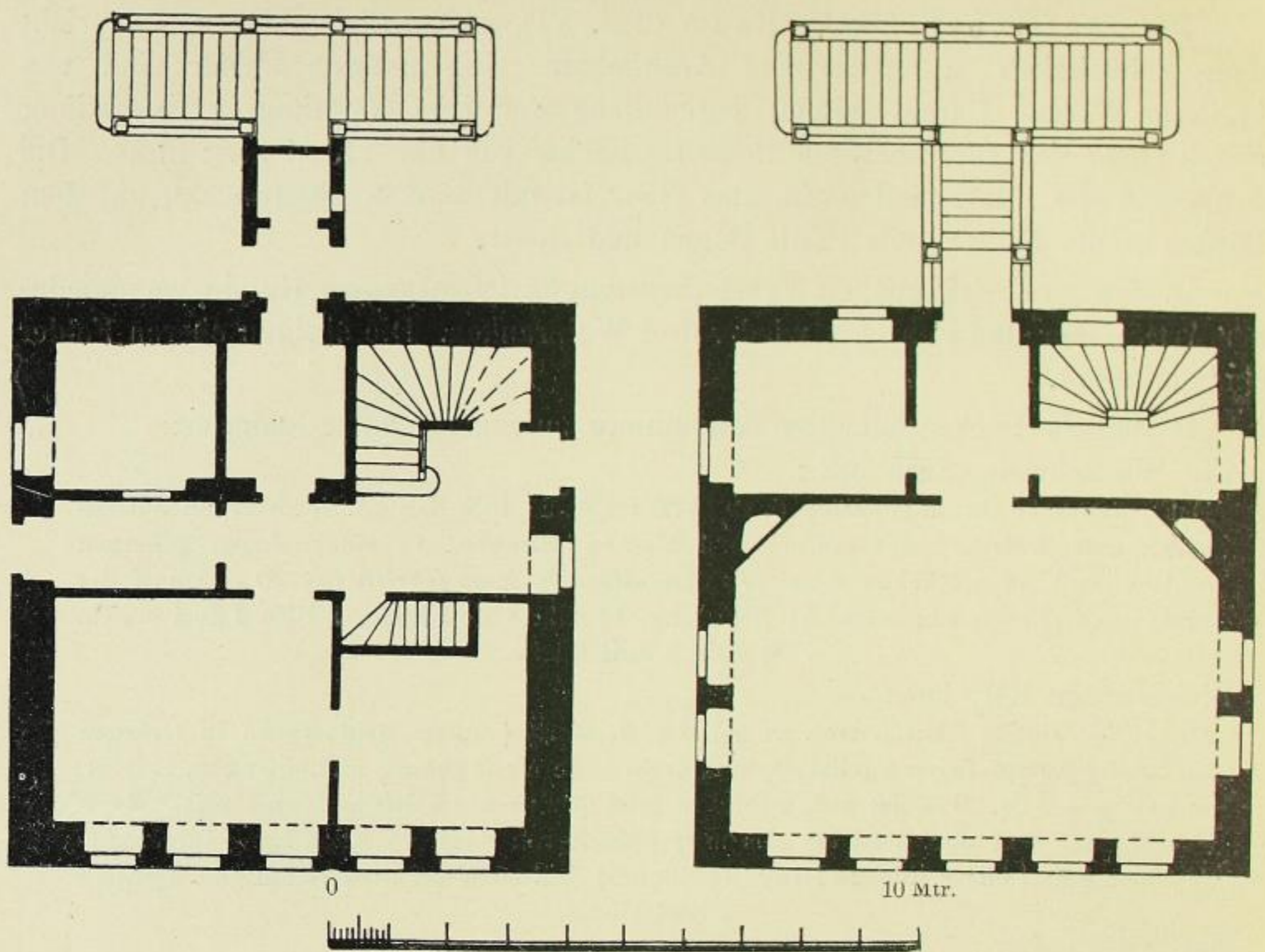
Fig. 153, 154. Spitzhaus, Grundriss der beiden Obergeschosse.
