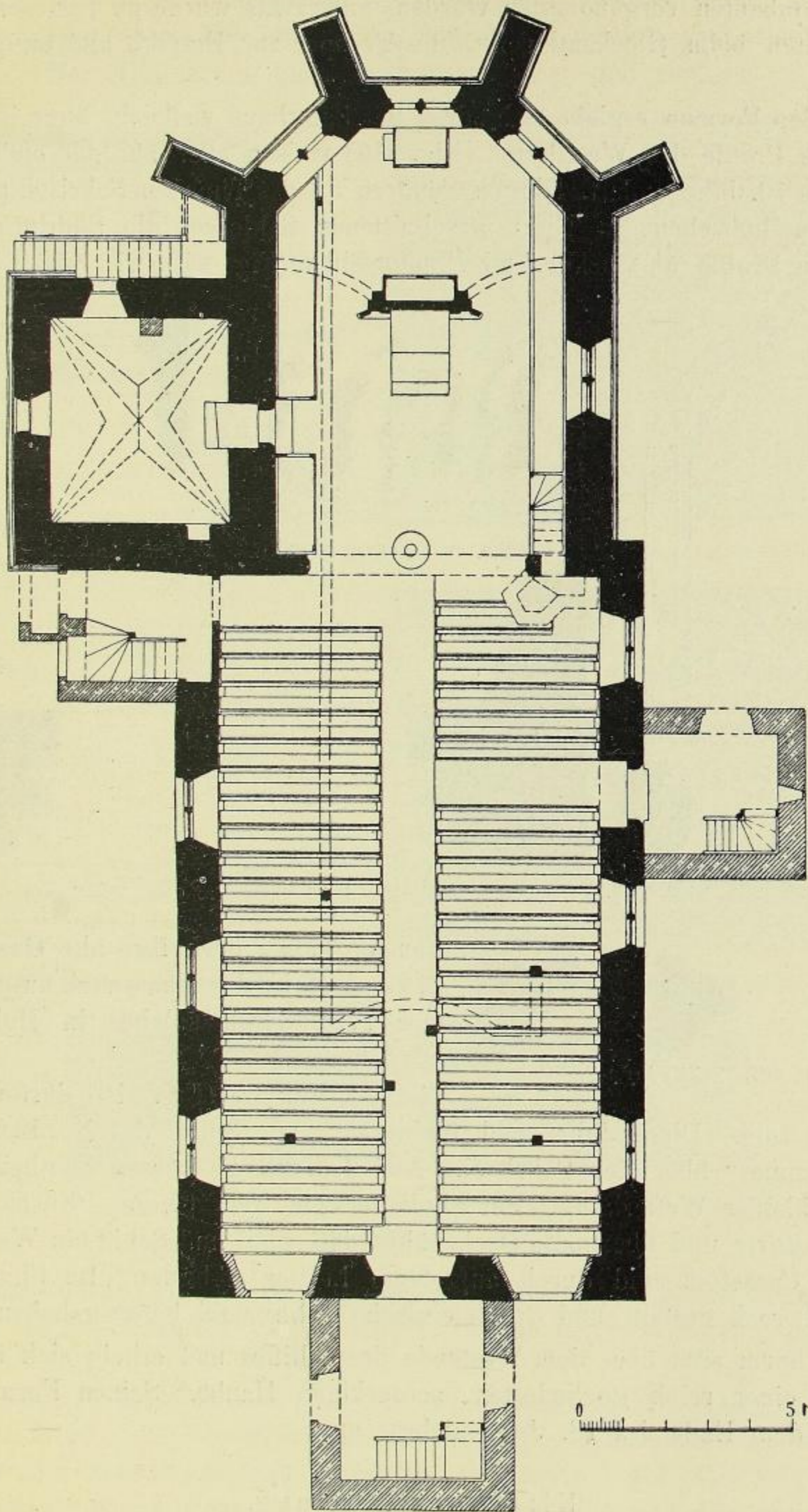
Fig. 211. Reichenberg, Grundriss der Kirche.
