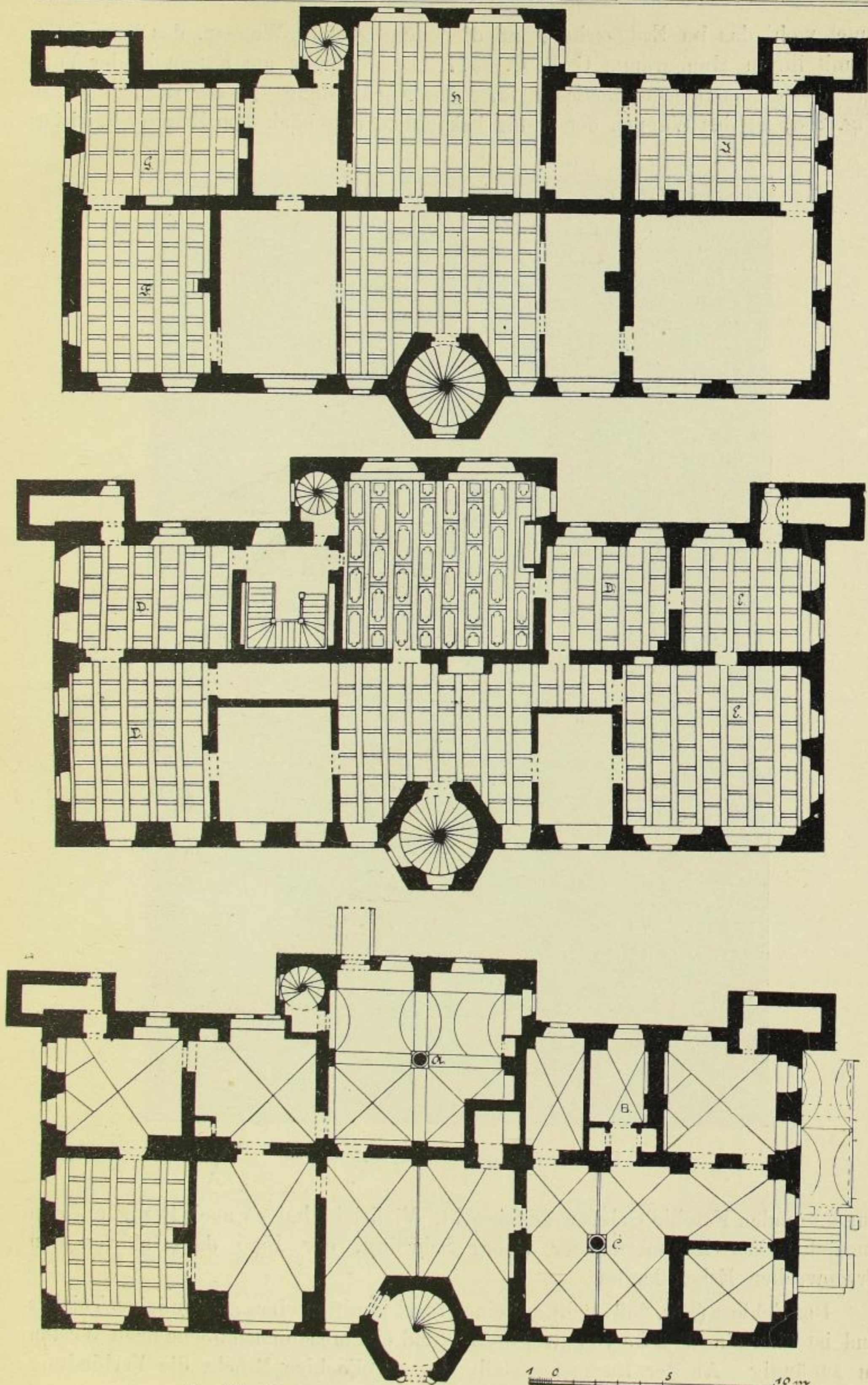
Fig. 234—236. Schönfeld, Schloss, Grundrisse der drei Geschosse.
