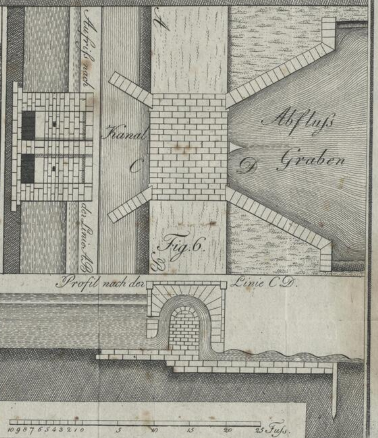
Woltman's Bauk. schiffb. Kanäle.
