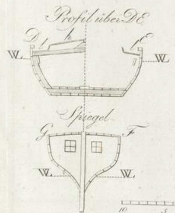
Fig. 26. Ein Ever auf der Niederelbe gebräuchlich.
