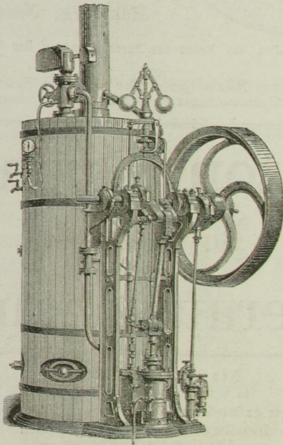
Vertikale Dampfmaschine am Kessel montirt.
