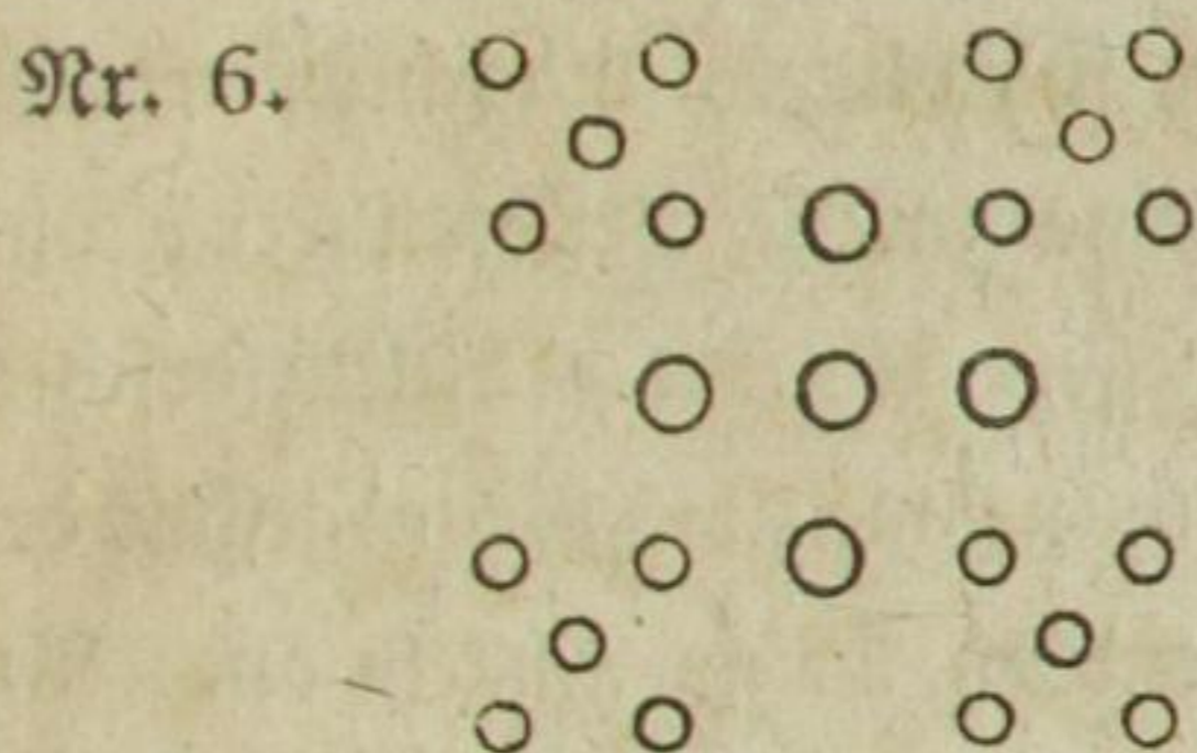
Zusammengetretene Gruppe von mehreren Braunbleyoxydato men.
