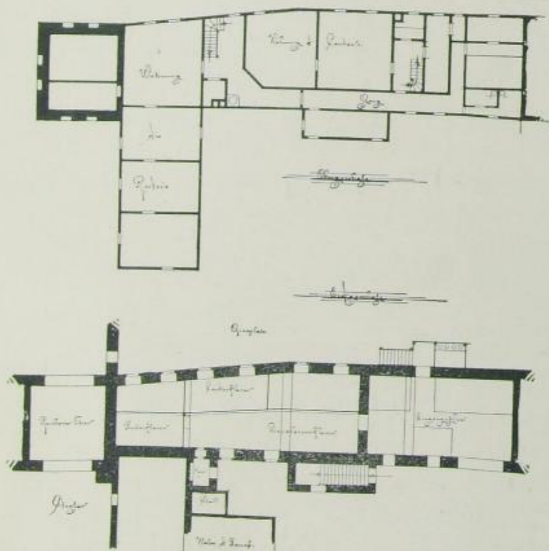
Grundriss dazu. (Die auf dem unteren Risse eingezeichneten durchgehenden schwachen, senkrechten Linien weisen auf den inneren Umbau 1826 hin.) (Vergleiche den Text Seite 50.)
