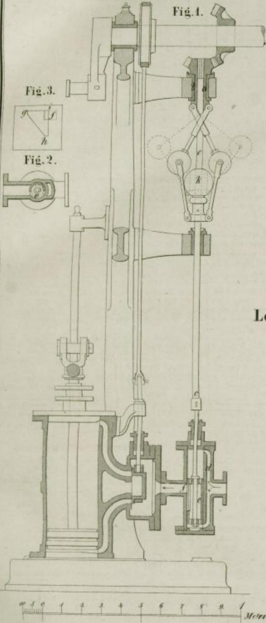
Maschine mit variabler Expansion von E. Paschke.
