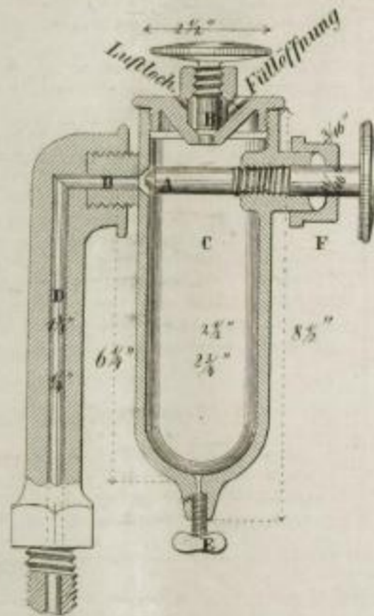
Schmiervorrichtung für Locomotiven-Steuerschieber.
