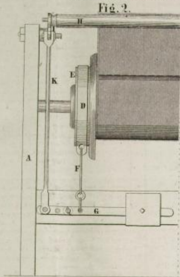
Schmiervorrichtung für Locomotiven-Steuerschieber.
