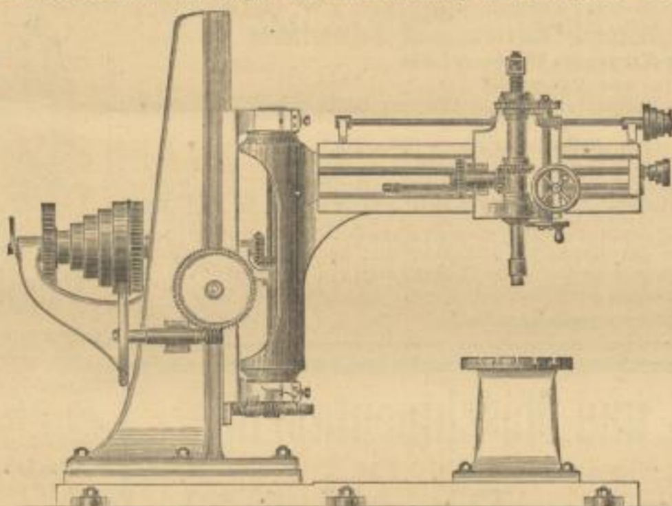
Radialbohrmaschine für Löcher bis 150 mm Durchmesser.
