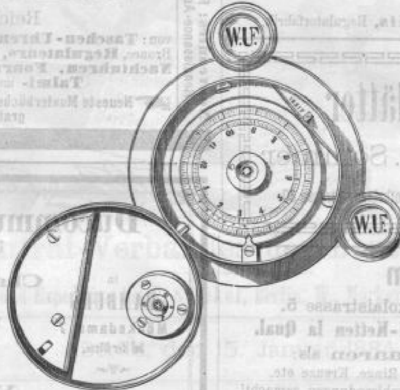
No. 3. Bürk's stationäre Control-Uhr.
