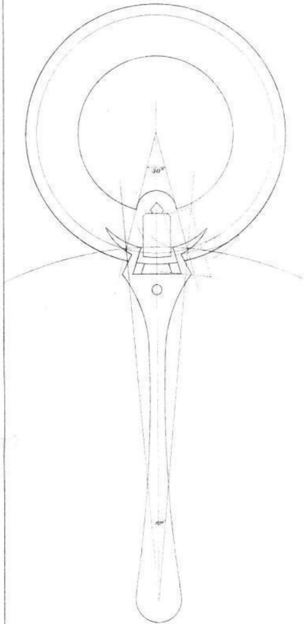
Ankerhemmung. F. Dencker, Hamburg.
