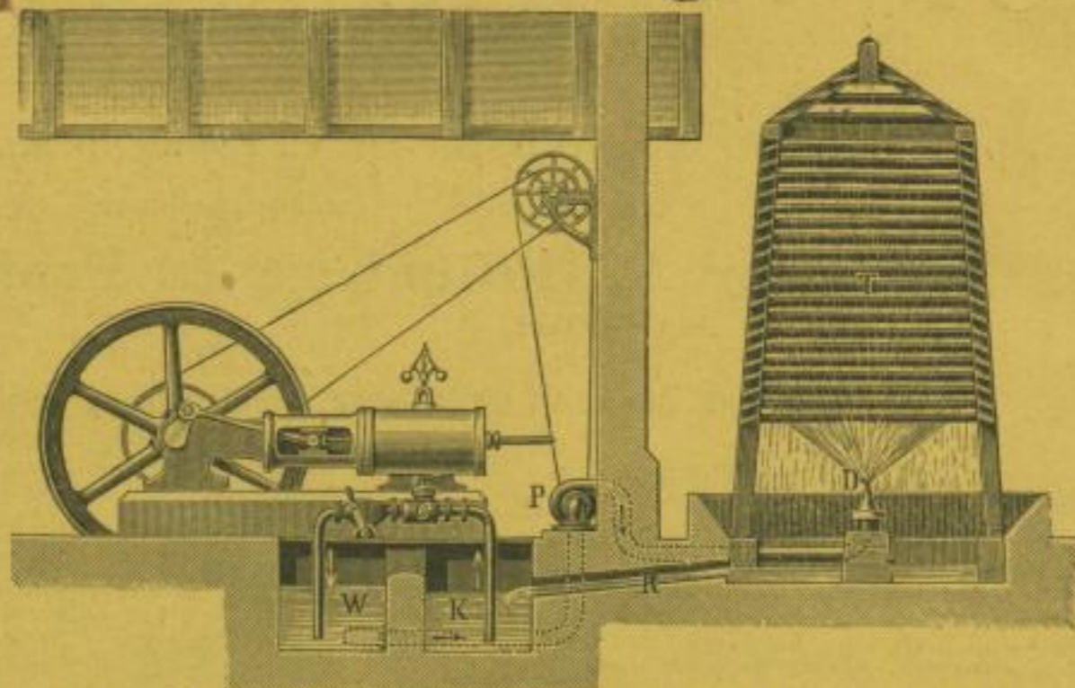
Condensations-Anlage mit Kühlung des gebrauchten Wassers durch Körting's Strahl-Condensator und Streudüsen.
