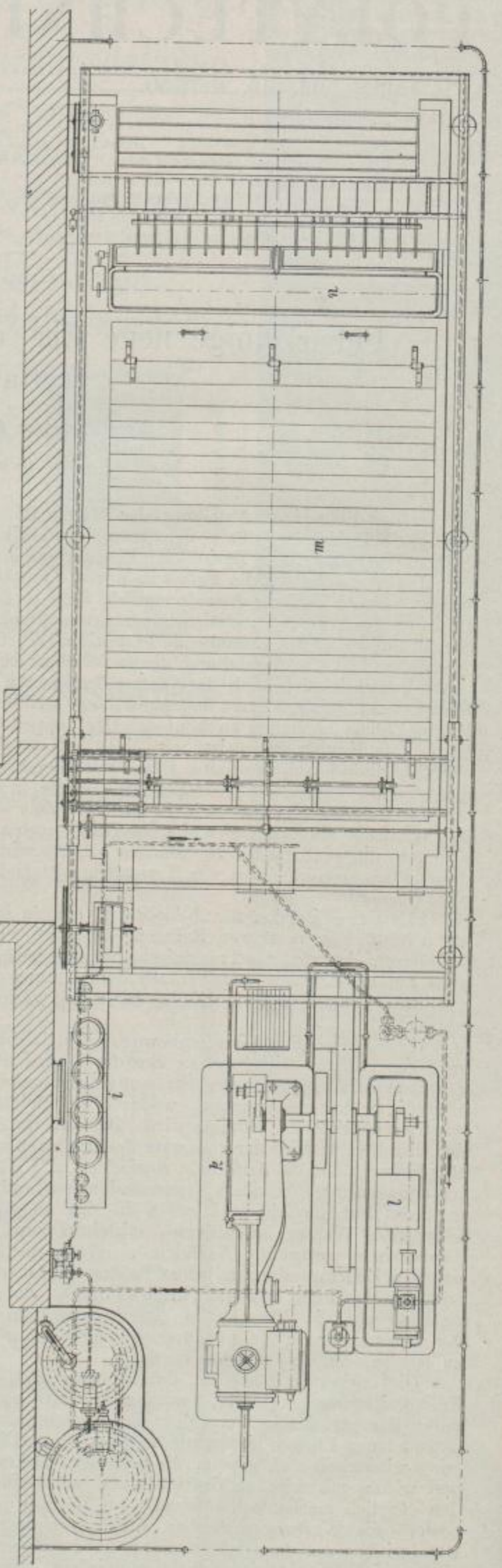
Eismaschine der Aktiengesellschaft der Maschinenfabriken von Escher, Wyss und Cie. in Zürich, Querschnitt.
