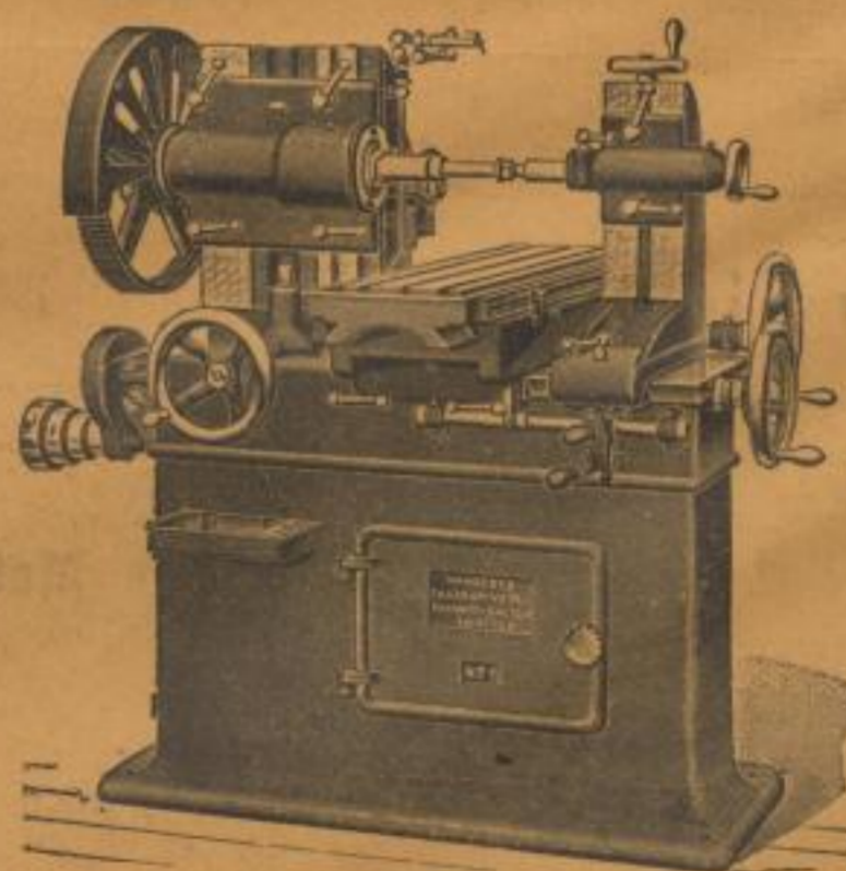
Planfräsmaschine No. 1.
