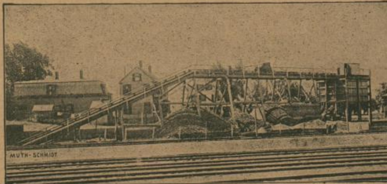
Gurtförderer mit autom. Materialverteiler für Beschickung eines Kohlenlagerplatzes.
