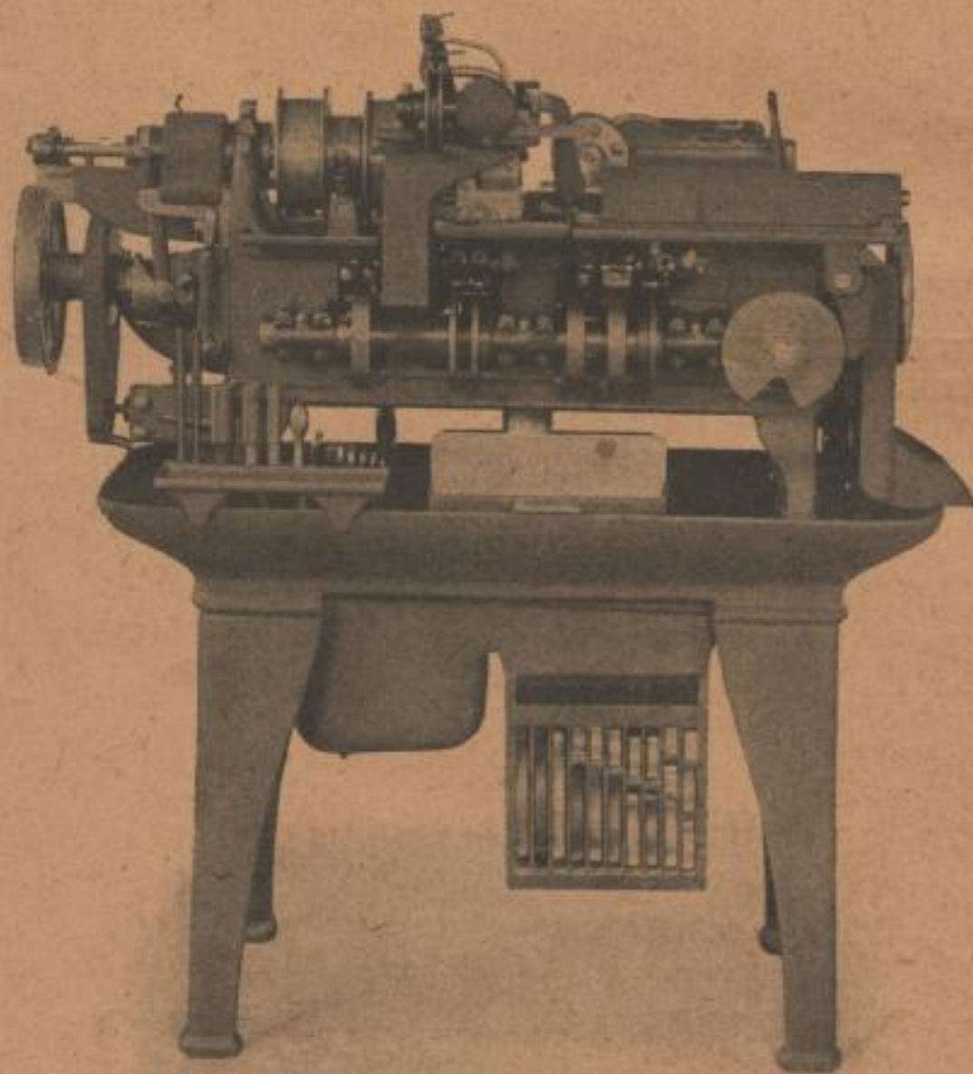
Präzisions-Schraubenautomat
