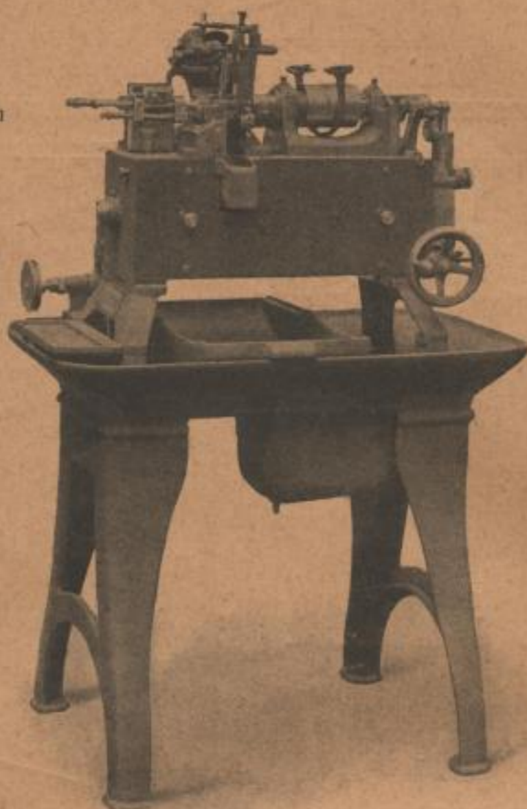
Präzisions-Schraubenautomat
