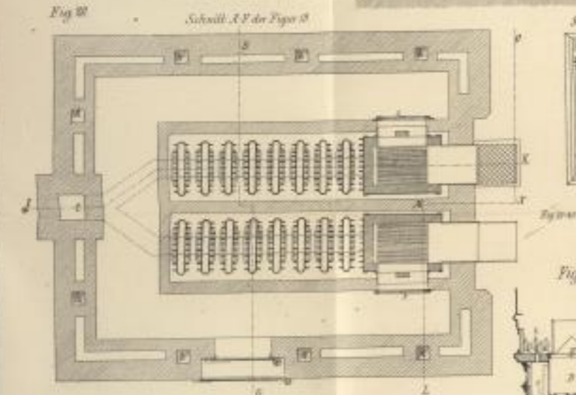
Krüger und Jussen's Ofen mit Marmormantel. (19-20)
