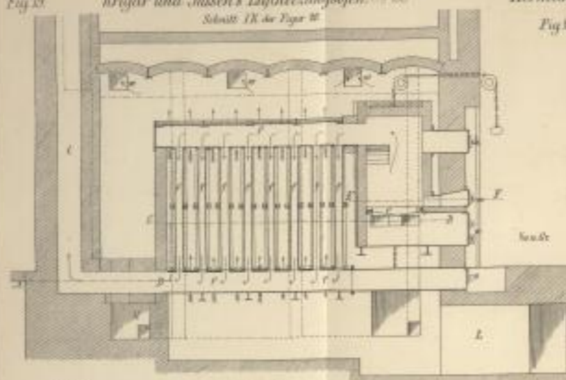
Fig. 27. Krüger und Jussen's Luftheizungsöfen. (17-18)
