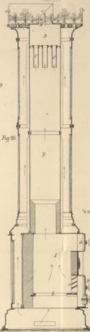
Fig. 27. Durchschnitt des Untertheils der Figur 27
