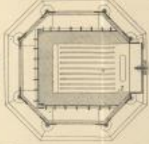
Fig. 27. Durchschnitt des Untertheils der Figur 27
