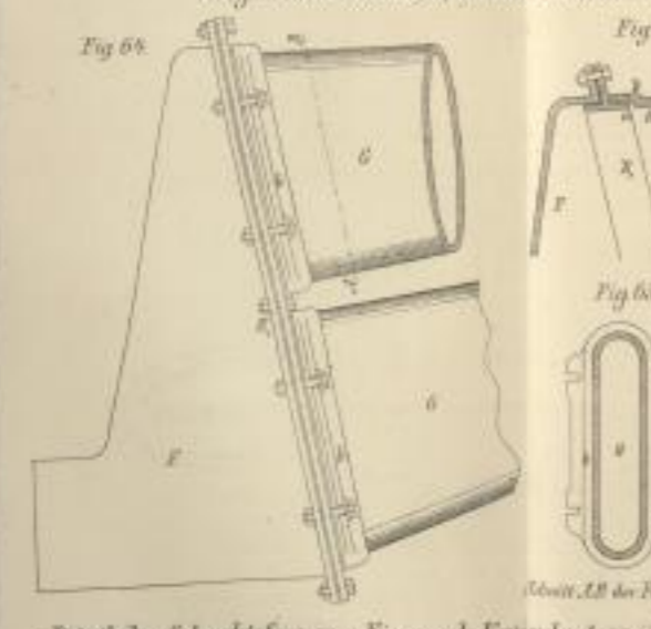
Detail des Schachtrofens vom Eisenerk Hüttenluthern. (21-22)
