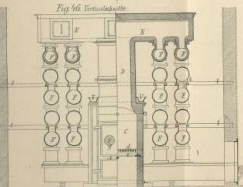
Kölling's Luftheizungsöfen (45-51)
