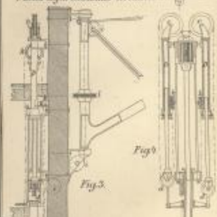
Stochnell's Gewandzähler (176-177)
