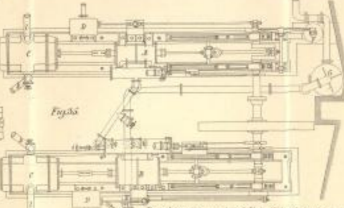
Bouchacourt und Dollé's Holzschrauben-Schneidmaschine (177)
