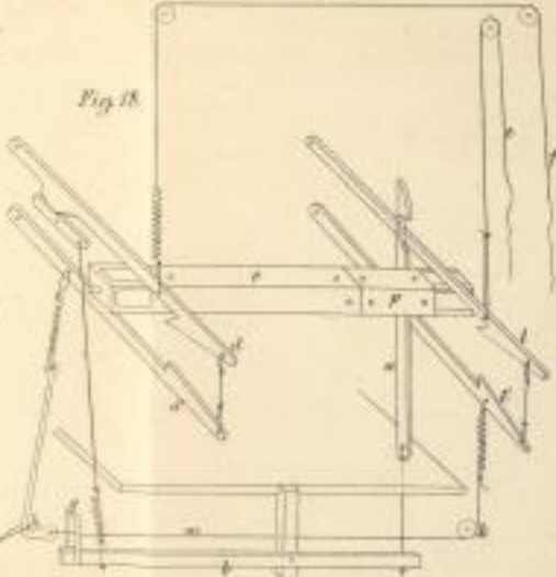
Asst's verbesserte Doppeljacquardmaschine (179)
