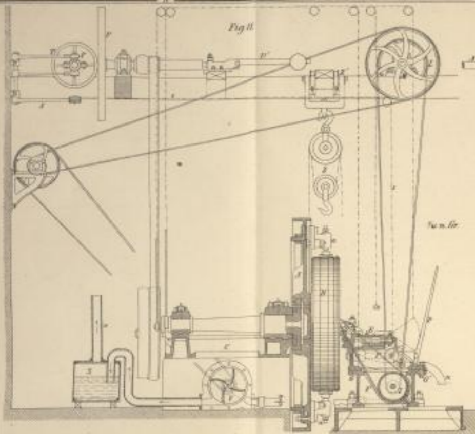
Royer's Maschine zum Zurechten der Mühlsteine (17-23)
