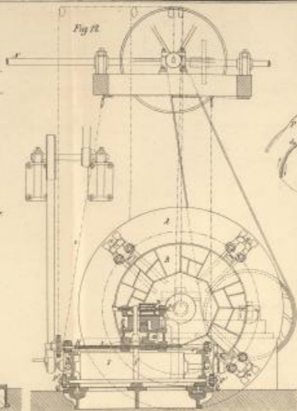
Goubet und Monroq's metallische Transmission (17-51)
