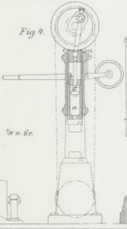
Chenot's pneumatische Hämmer. (3-5)
