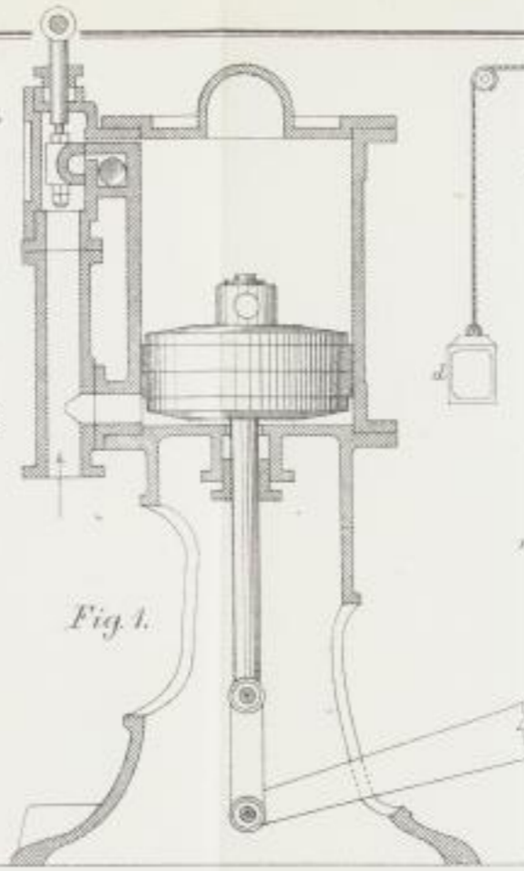
Chenot's pneumatische Hämmer. (3-5)
