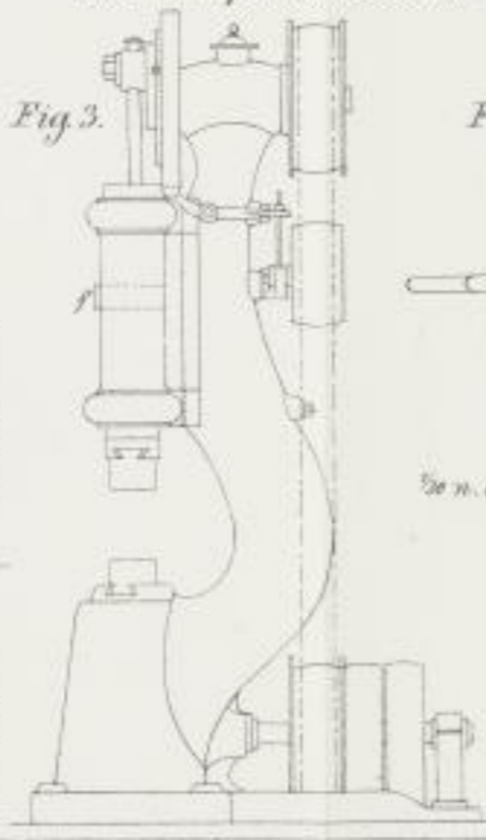
Chenot's pneumatische Hämmer. (3-5)
