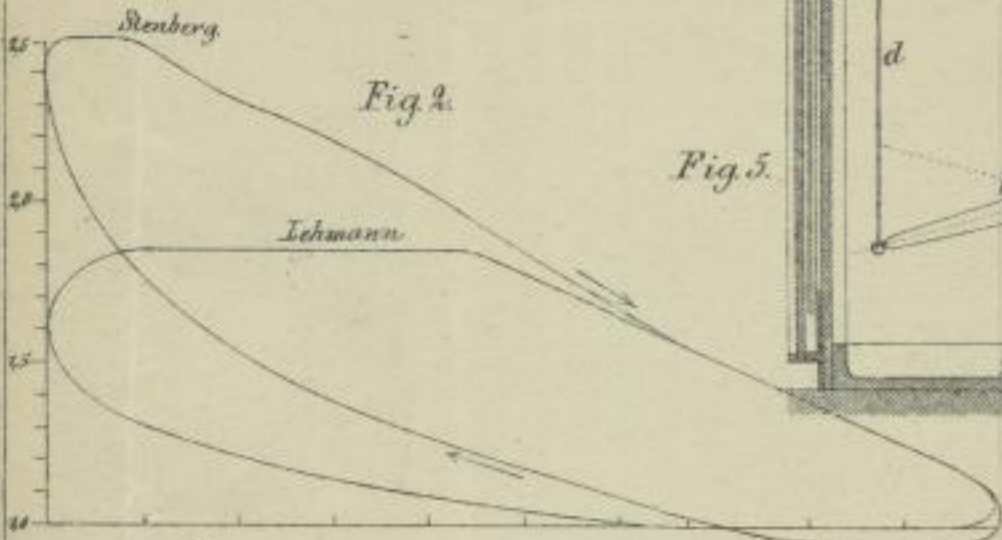
Stenberg's Heißluftmaschine. (1 u. 2)
