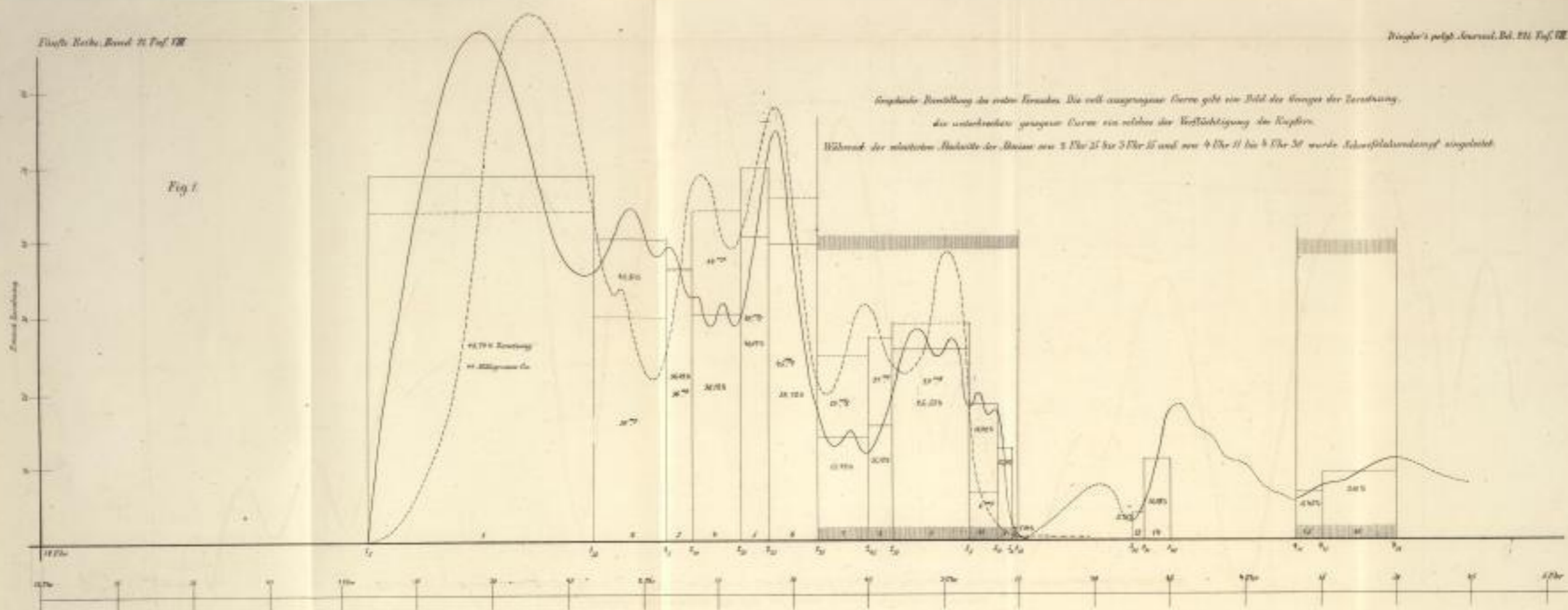
D' Jürsch: Beiträge zur Kenntnis des Bunsen'schen Processes der Chloräthylherstellung (Fig. 1 u. 2)
