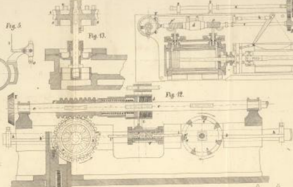
Schalldrucktelegraph (19)
