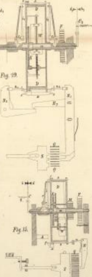
Schalldrucktelegraph (19)
