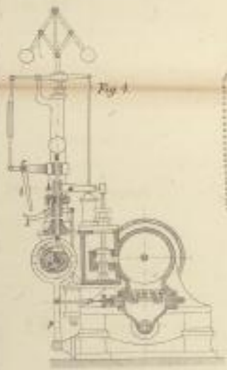
Kollet's Ventilsteuerung (1)
