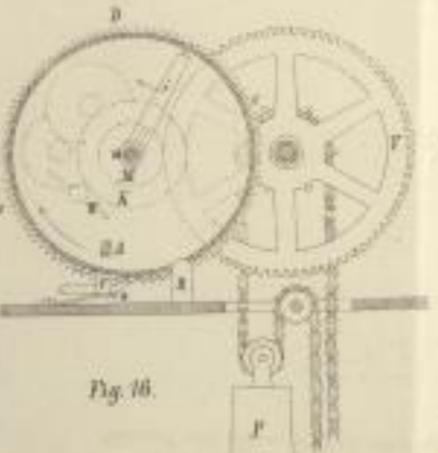
Siemens und Halske's automatische Stromsender für telegraphische Schnellschrift. (16-19)
