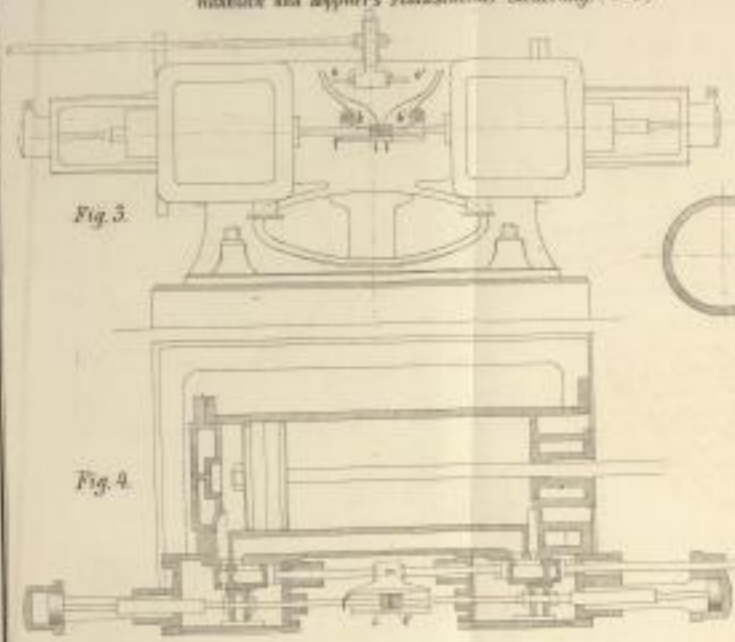
Kollet's Ventilsteuerung (1)
