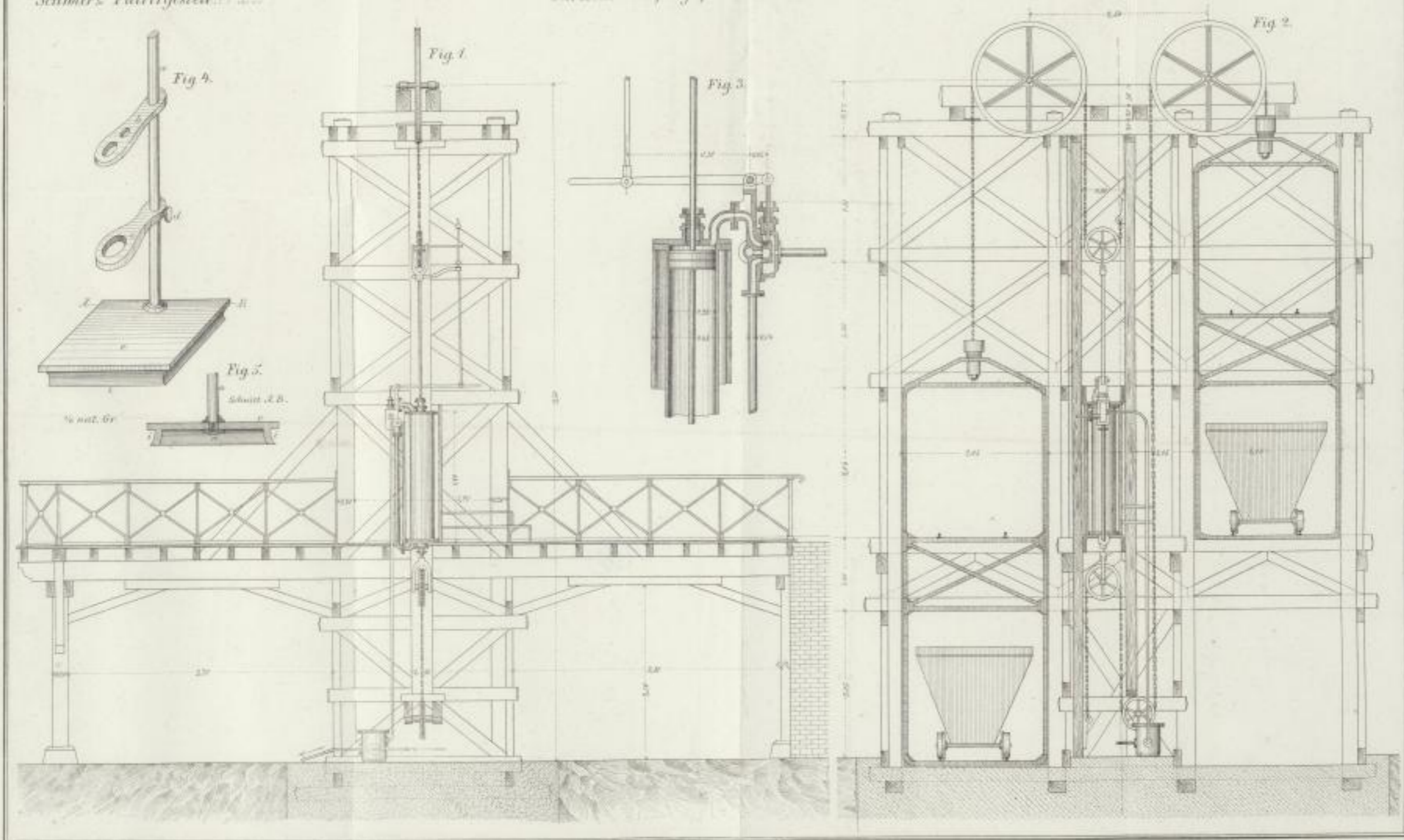
Chrétien's Aufzug für Coaksöfen (17 u. 53)
