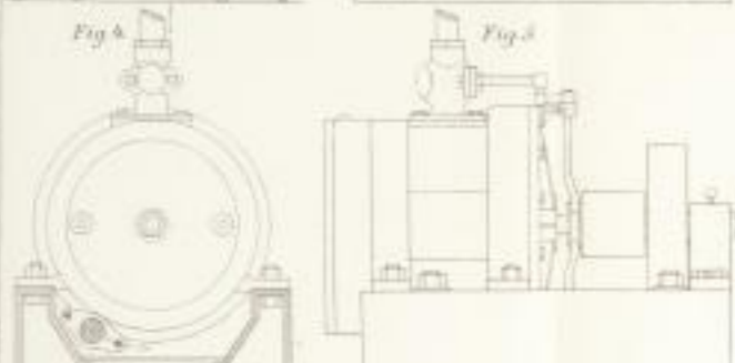
Egli's Dampfschnittapparat
