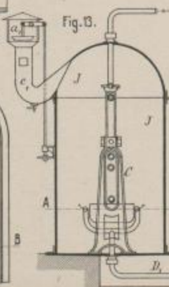
Schnitt A B von Fig. 13.
