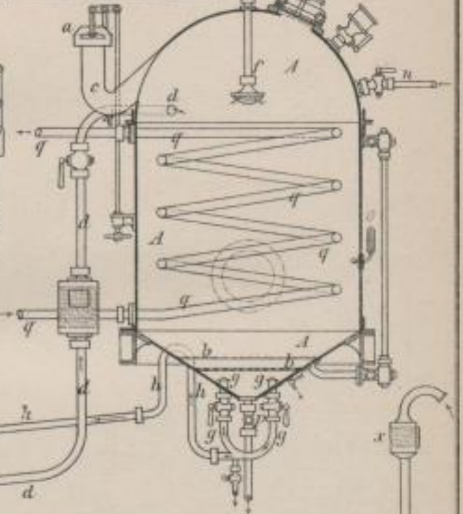
Apparat zum Sterilisiren und Kühlen der Bierwürze. (12-14)
