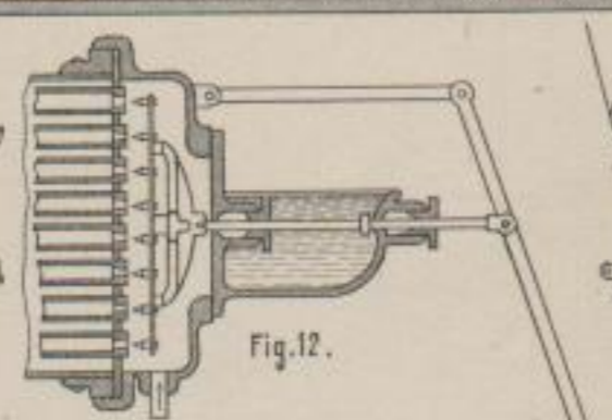
Yaryan-Verdampfapparat. (12 u. 13)
