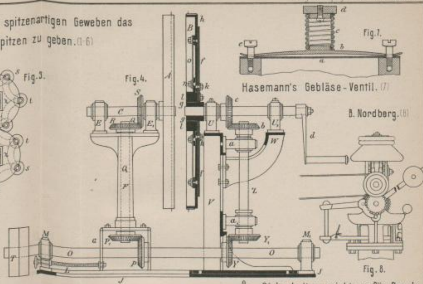
Sicherheitsvorrichtung für Regulatoren. (8)
