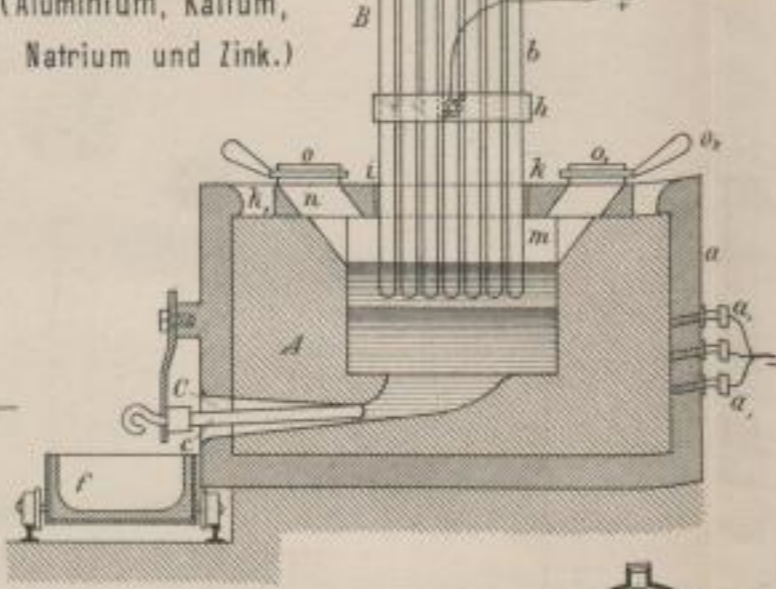
Fig. 3. Herstellung von Aluminiumbronze der metallurg. Gesellschaft in Neuenhausen.
