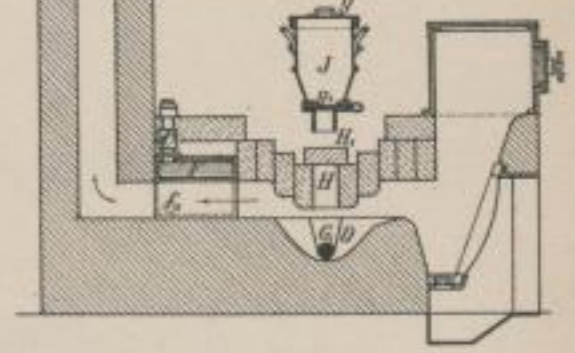
Fig. 4. Thompson und White's Reduktionsofen für Aluminium.
