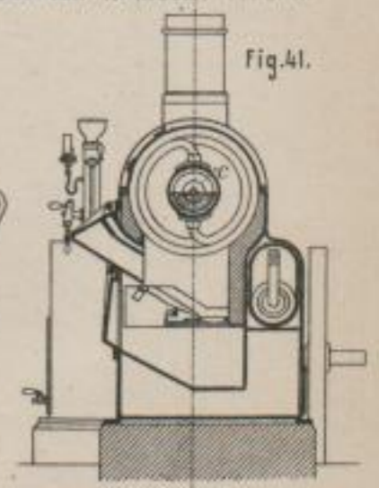
Rotirender Kessel von A. Musil. (40 u. 41)
