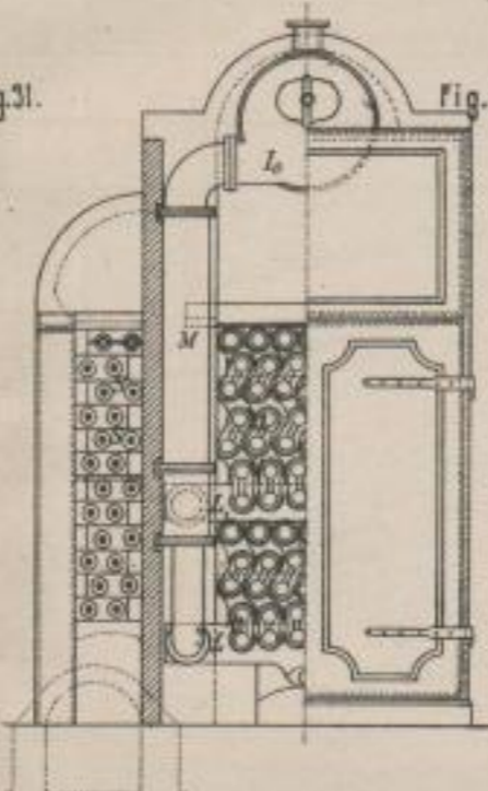
H. Gollner: Ueber Dampfkessel. (Fig. 30-41)
