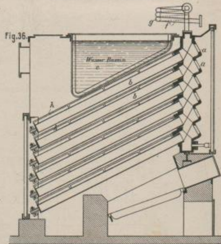
Dampfkessel der Leipziger Röhrendampf- kesselfabrik Breda u. Co. (36 u. 37)
