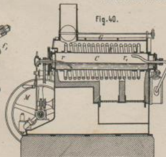
Rotirender Kessel von A. Musil. (40 u. 41)
