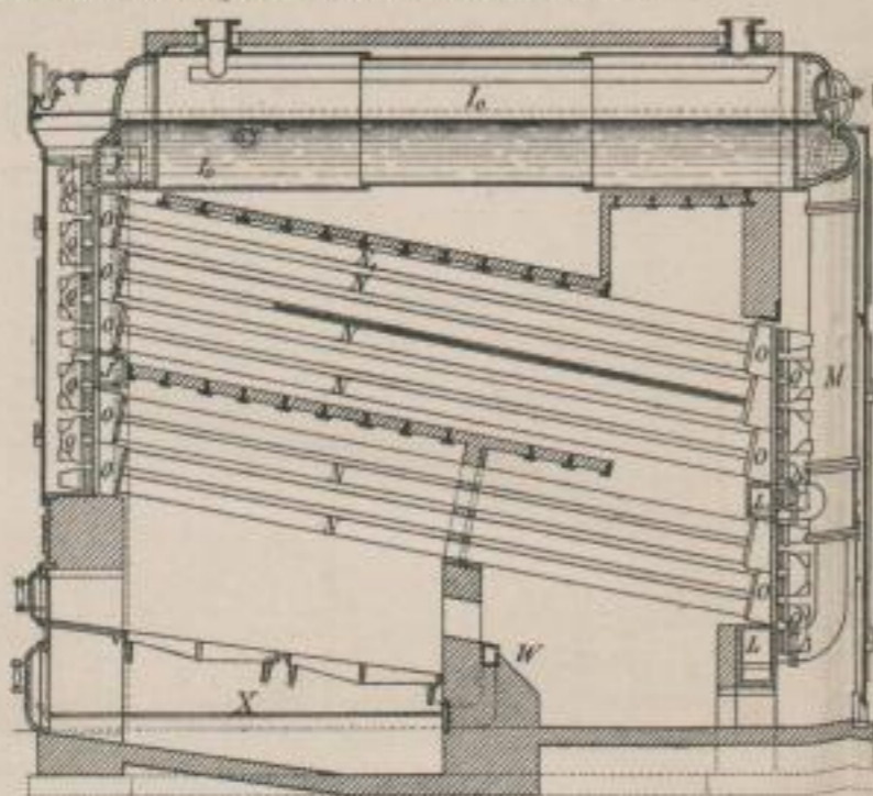
H. Rittner's Gliederkessel. (34 u. 35)
