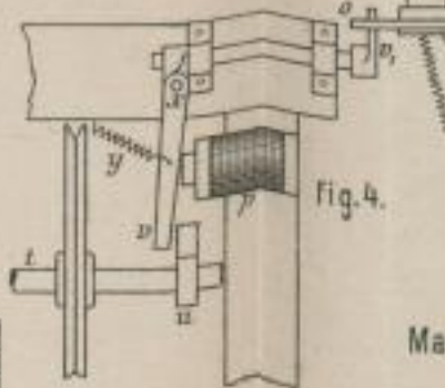
Maschine zur Anfertigung von Kantillen. (1-4)
