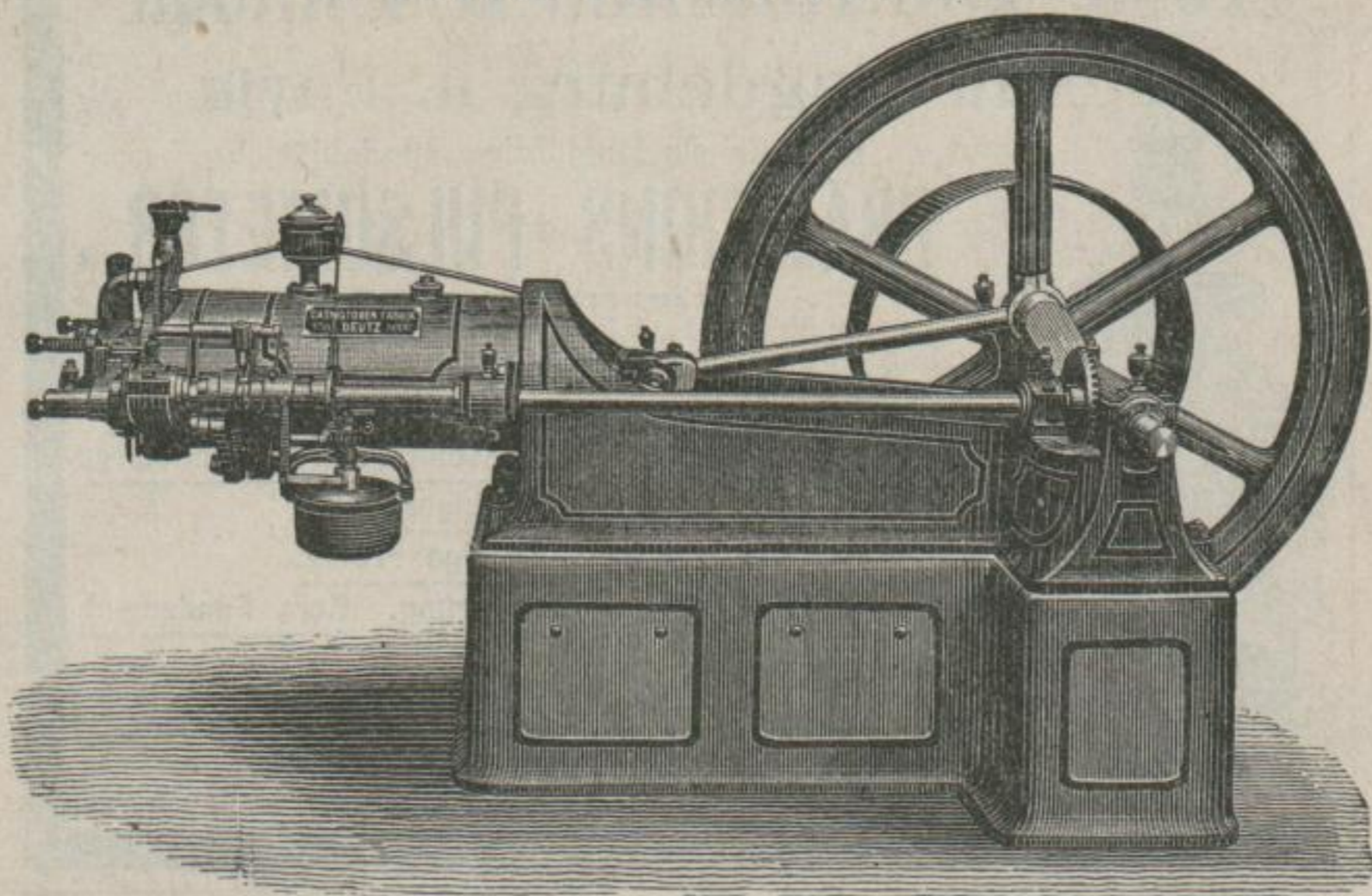
Otto's neuer Motor. (Durch Patente geschützt.)
