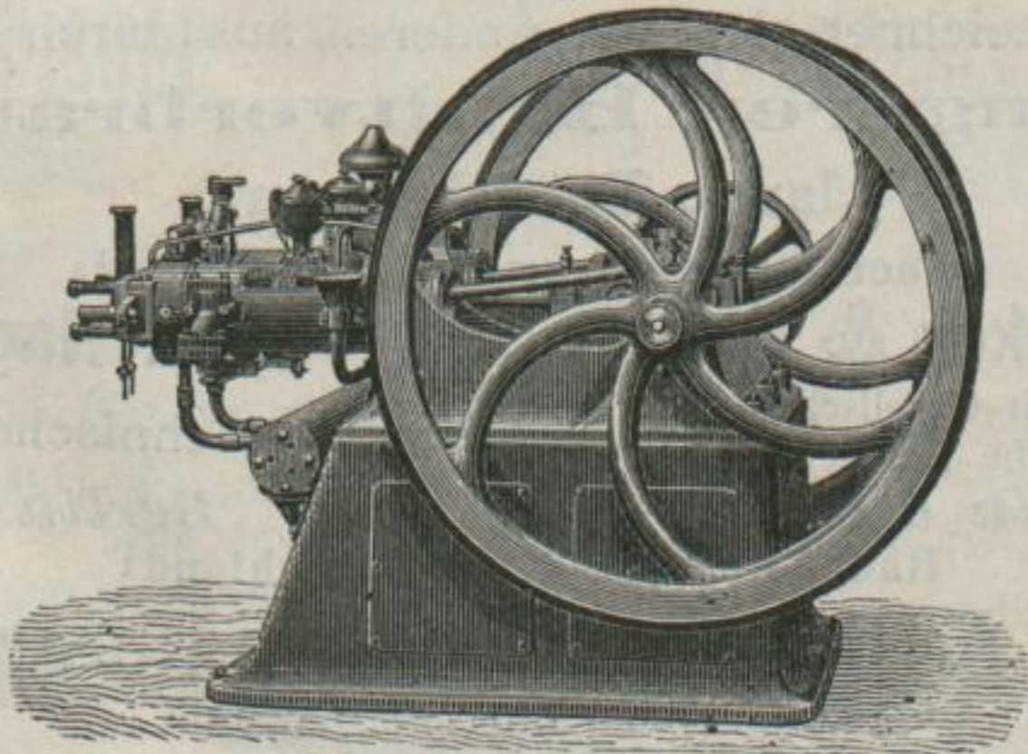
Zwillingsmotor.
