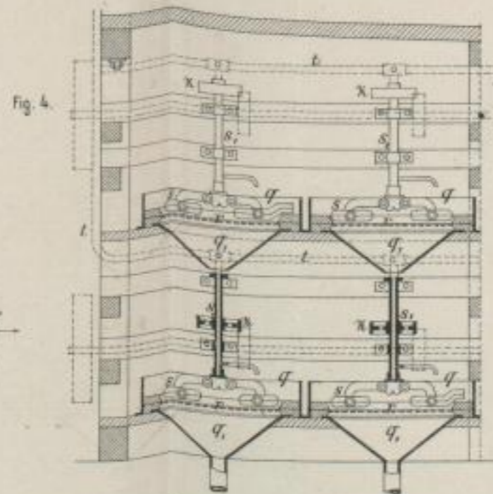
L. v. Wagner und A. Gillitzer's Siebapparat zur Stärkefabrikation. (4)
