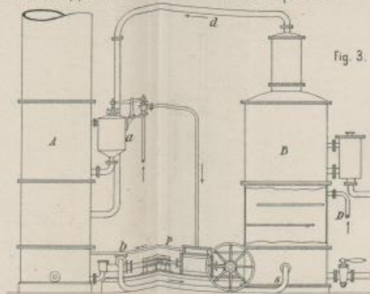
J. Höper's Verdunstapparat mittels überhitzten Dampfes. (3)
