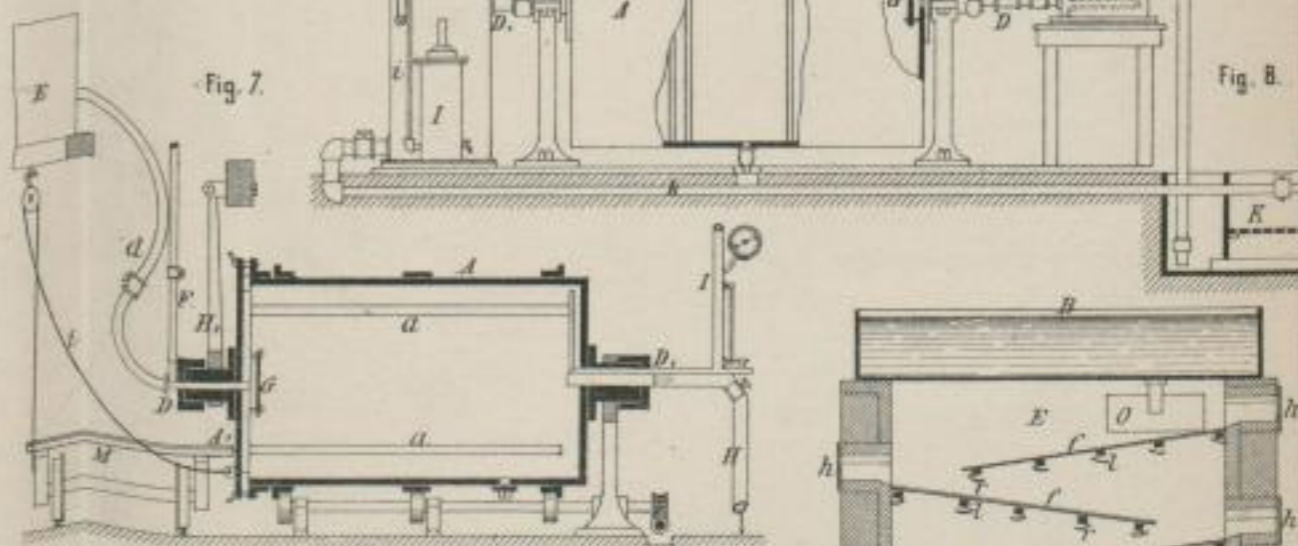
R. Schneider's Abdampföfen. (9-11)
