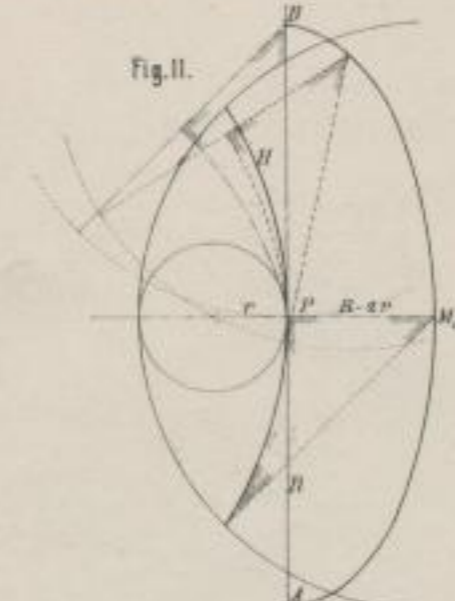
G. Oldenburger's Universal-Kegelschnittzeichner. (18)
