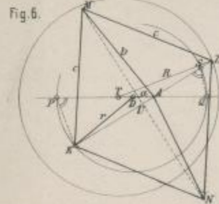
Epicyclisches und hypocyclisches Rollsystem. (10 u. 11)
