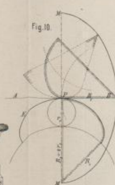
G. Oldenburger's Universal-Kegelschnittzeichner. (18)
