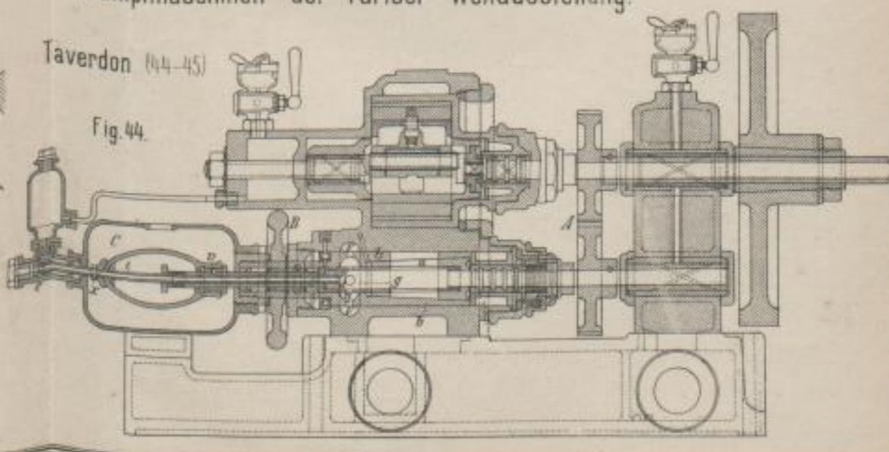
"Dampfmaschinen der Pariser Weltausstellung.
