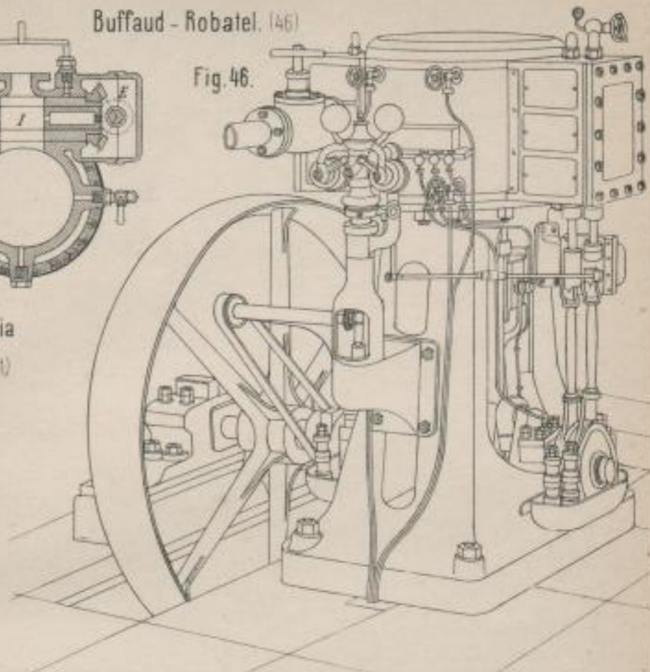
"Dampfmaschinen der Pariser Weltausstellung.
