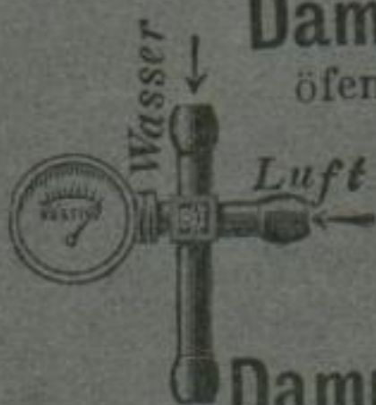
Wasserstrahl-Luftpumpe.
