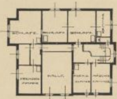
OBERGESCHOSS
